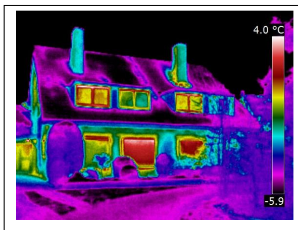
Voorbeelden van ontbrekend isolatiemateriaal in het dakbeschoot en bij de schoorstenen
