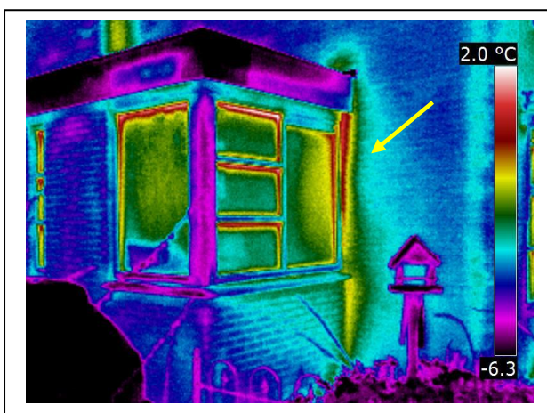
Voorbeeld van energieverliezen bij de aansluiting met het originele woonhuis
