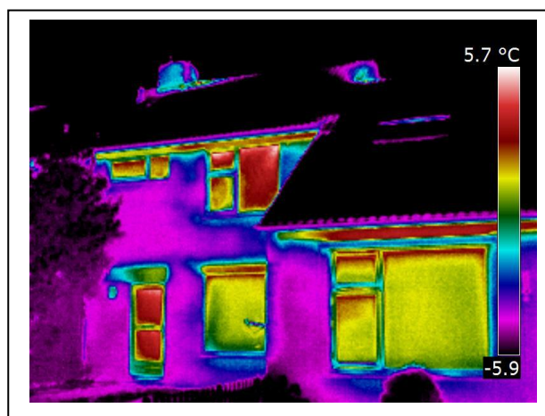
Woningen met kozijnen met enkelglas op de 1 ste verdieping
