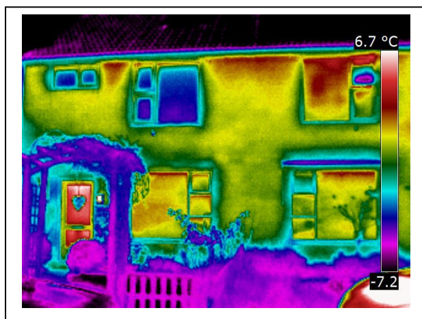
Voorbeelden van woningen waarbij enkel glas op de 1 ste verdieping is vervangen door HR-glas.
