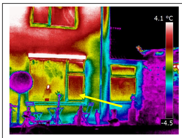
Woning met onder meer warmteverlies via de woning vanuit de beter geïsoleerde aanbouw.
