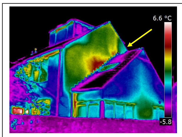
Voorbeeld van energielekken bij de aansluiting uitbouw en gevel.
