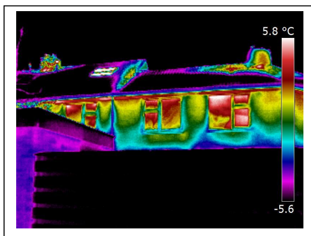
Woningen met kozijnen met enkelglas op de 1 ste verdieping
