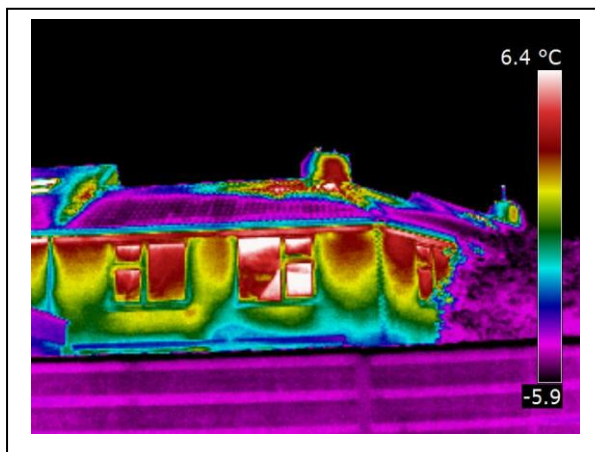
Voorbeeld van een dak met zwakke plekken rond de schoorsteen en langs de nok
