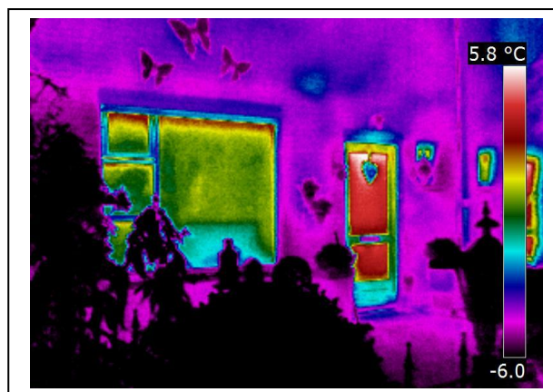
Woning met een enkelglas in de voordeur en met standaard dubbelglas in het woonvertrek.
