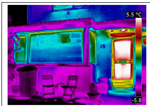
Woning met een enkelglas in de voordeur en met HR- glas in de uitbouw.
