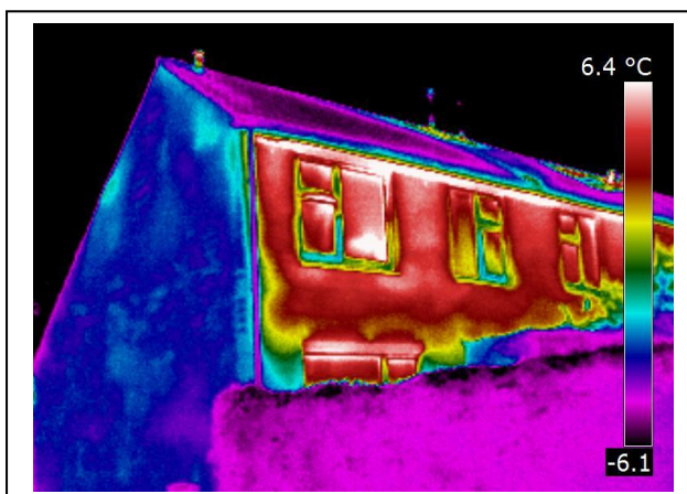
Voorbeeld van een geïsoleerde kopgevel en ongeïsoleerde achtergevels
