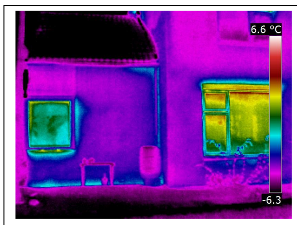
Gelijkwaardig geïsoleerde uitbouw maar met een betere kwaliteit isolatieglas.
