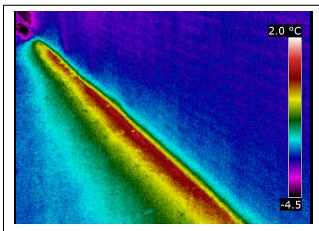
Voorbeeld van luchtlekken bij de aansluiting bij begane grondvloer met de gevel.
