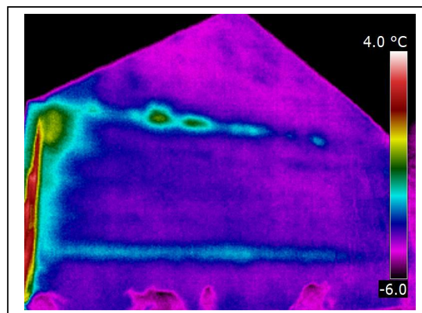
Voorbeeld van energieverliezen via luchtlekken de aansluiting verdiepingsvloer en de gevel.
