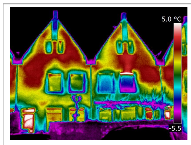
Voorbeelden van slecht geïsoleerde gevels in het westelijk deel van De Noordbuurt
